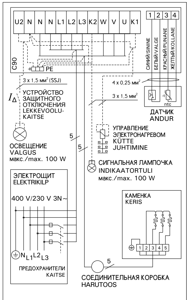
Рисунок 12б. Электромонтаж пульты управления C90 и каменки BC-E (подключение в 3-фазной сети)
