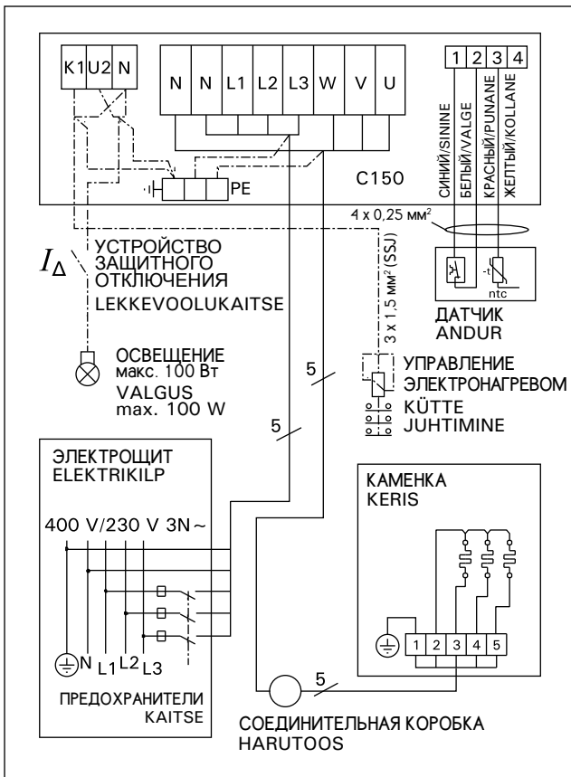
Рисунок 12а. Электромонтаж пульты управления C150 и каменки BC-E (подключение в 3-фазной сети)
